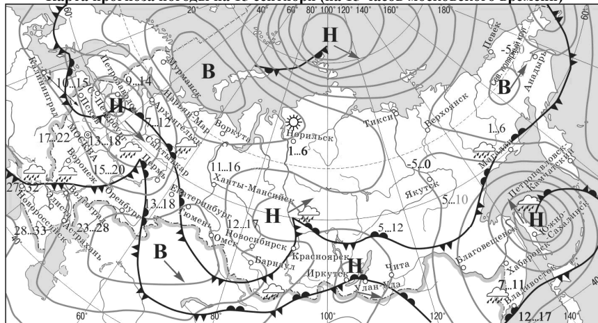
Карта прогноза погоды на 15 сентября (на 15 часов московского времени)
